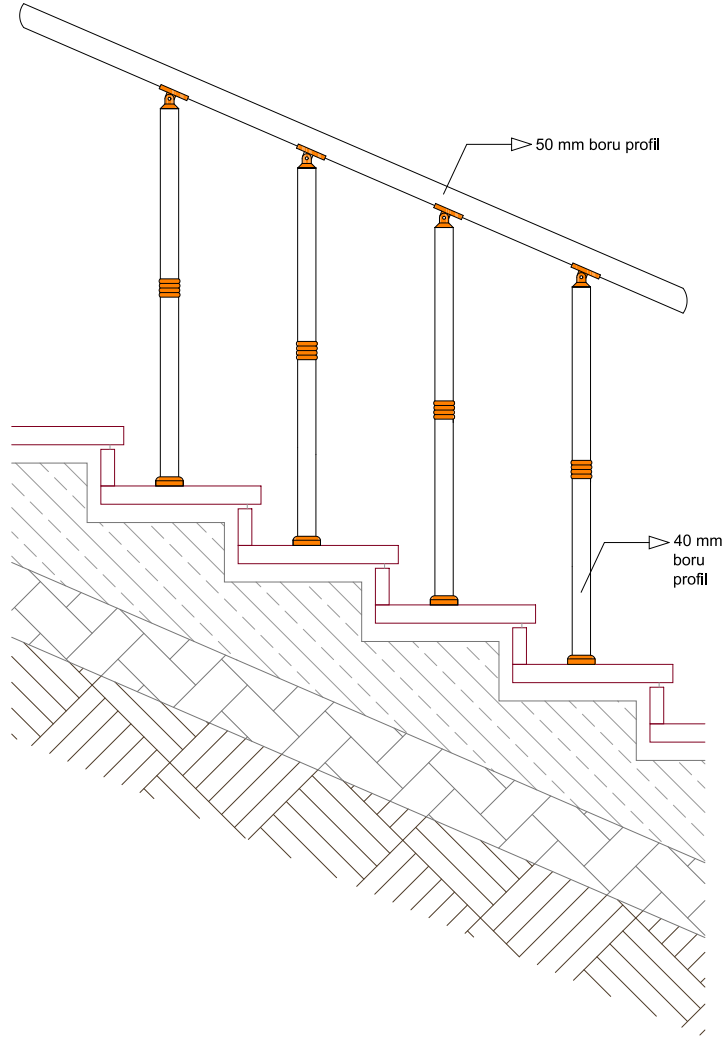
Camsız Dekorlu Korkuluk (Her Basamağa Bir Dikme,Dikmeler Döşemeye Üstten Bağlı)
