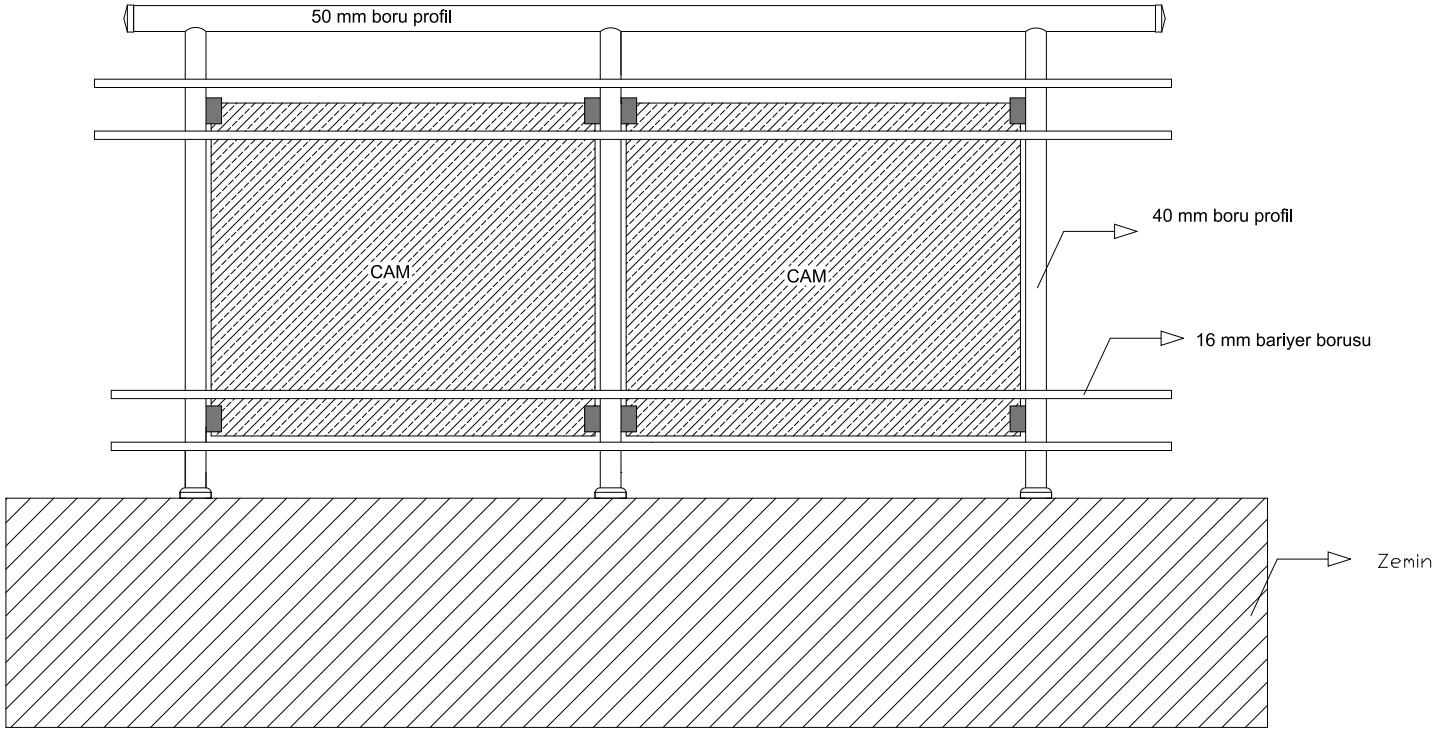
Camlı ve Bariyerli Korkuluk (Döşemeler Üstüne Üstten Bağlı Yatay 4 bariyerli)
