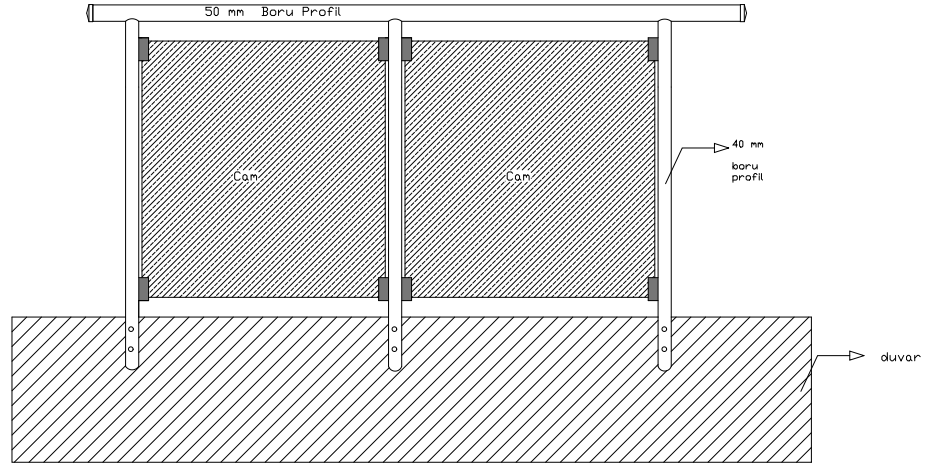
Camlı Korkuluk (Dikmeler Döşemeye Yandan Bağlı)
