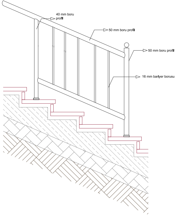
Camsız Korkuluk (DüŖey Bariyerli, Dikmeler DöŖemeye Üstten Bağlı)
