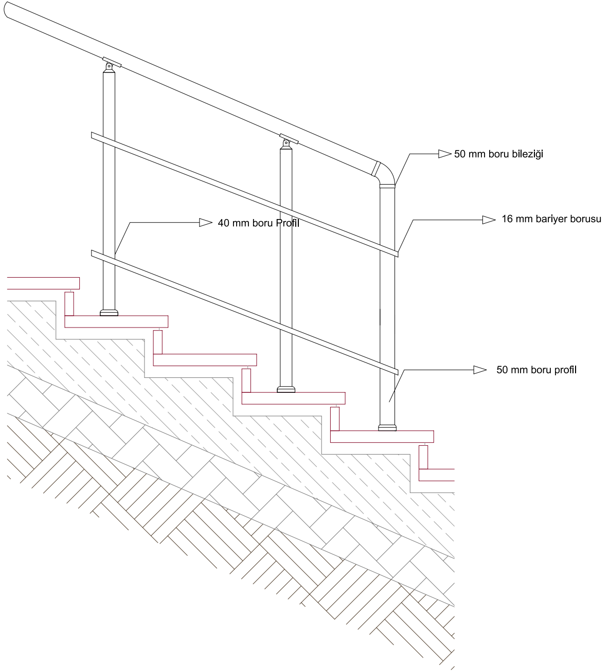
Camsız Korkuluk (Yatay İki Bariyerli, Dikmeler Döşemeye Üstten Bağlı)
