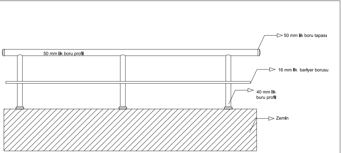
Parapet Üstü Korkuluk (Dikmeler Döşemeye Üstten Bağlı Tek Bariyerli)
