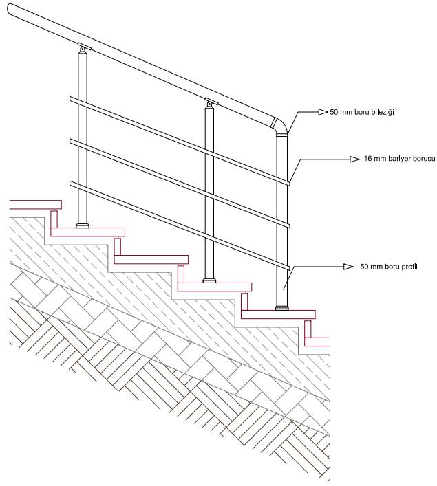
Camsız Korkuluk (Yatay Üç Bariyerli, Dikmeler Döşemeye Üstten Bağlı)
